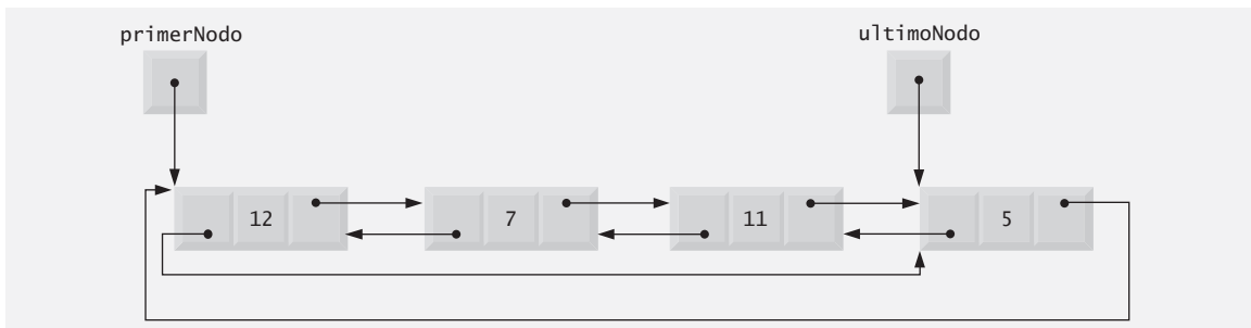
Figura 24.12 | Lista circular, doblemente enlazada.
