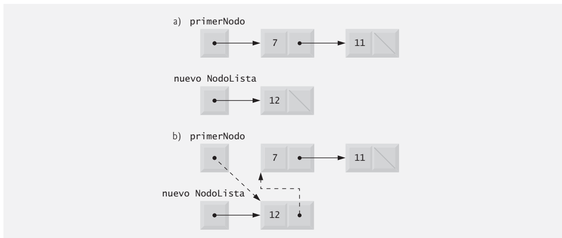
Figura 24.6 | La operación InsertarAlFrente.
