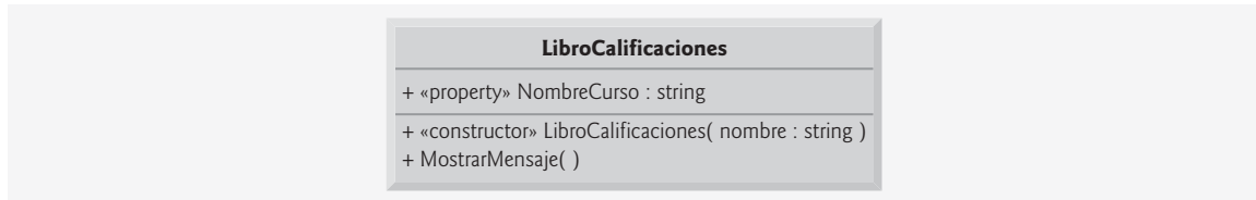
Figura 4.14 | Diagrama de clases de UML donde se indica que la clase LibroCalificaciones tiene un constructor con el parámetro Nombre del tipo string .
